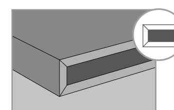
"MONOLITE" 3/4 FRAME Supporto in multistrato per l'installazione di tasselli a scomparsa. Open Unit for hidden fixing
